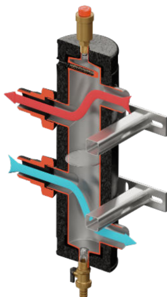
Sprzęgło hydrauliczne pionowe SHE-PRO
