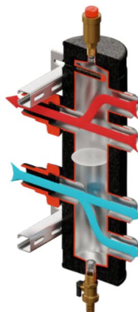
Sprzęgło hydrauliczne pionowe SHE-PRO 2K
