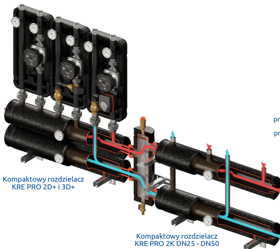
KRE PRO oddzielenie ciepłej i zimnej wody - izolacja EPP
