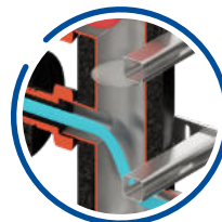
SHE-PRO przyłącza gwintowane DN 32 i 50 przyłącza kotłownicze DN65 i 80
