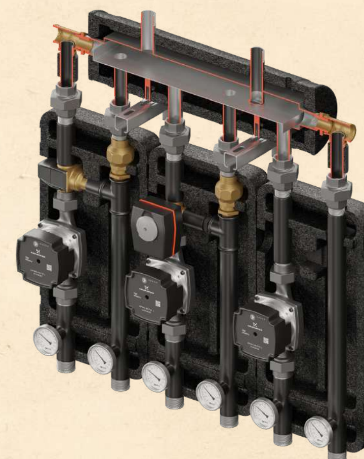
Zestaw mieszający Eskadra PRO 3D
