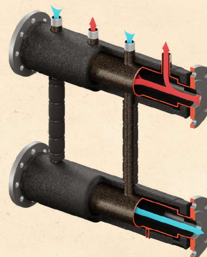
Kompaktowy rozdzielacz KR& PRO 2D
