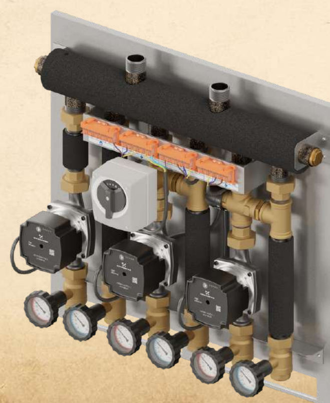
Zestaw mieszający Szwadron PRO 3D
