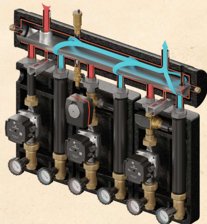
Zestaw mieszający Kompania 3D PRO
