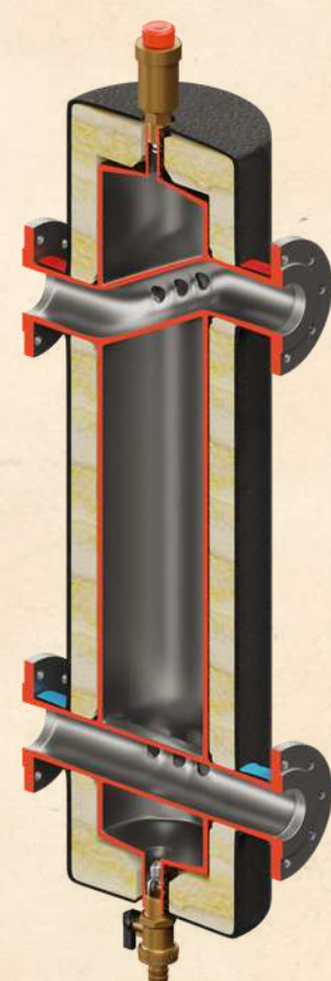
Sprzęgło hydrauliczne SH& CD
