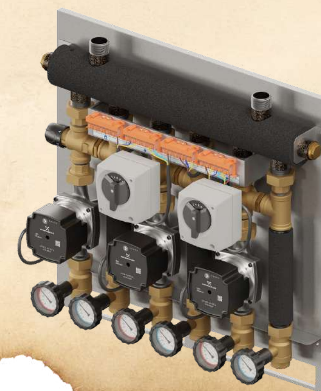
Zestaw mieszający Eskadra PRO 3D
