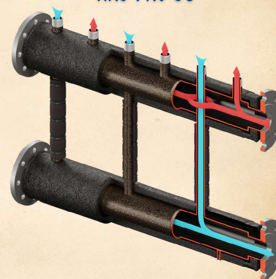
Kompaktowy rozdzielacz KR& PRO 3D
