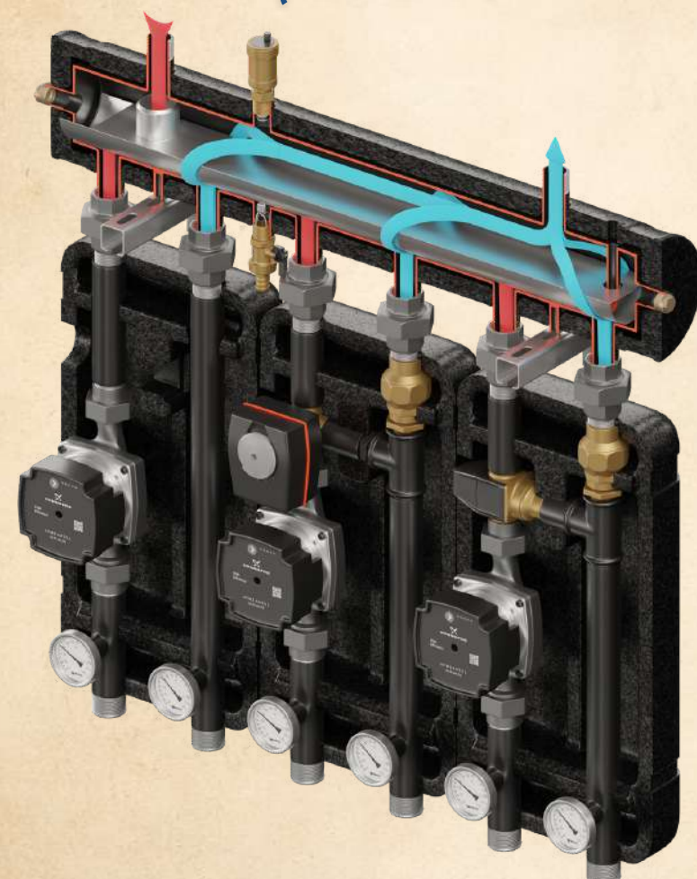
Zestaw mieszający Kompania 3D
