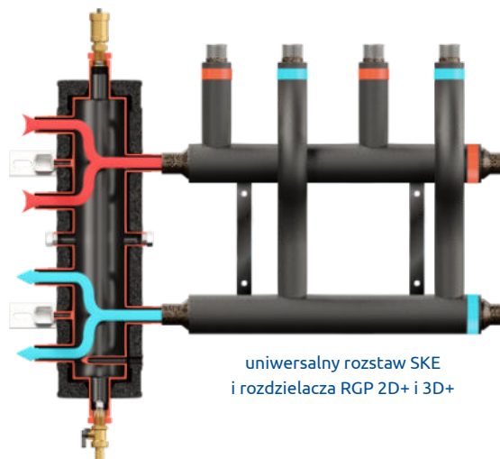
2 źródła ciepła + SKE 2D
