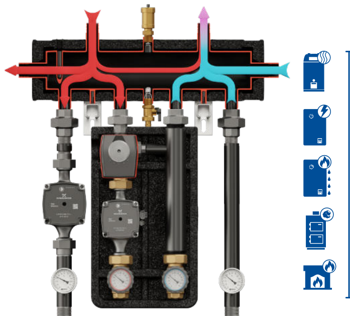
Prawidłowe podłączenie grupy pompowej z SKE 2D+
