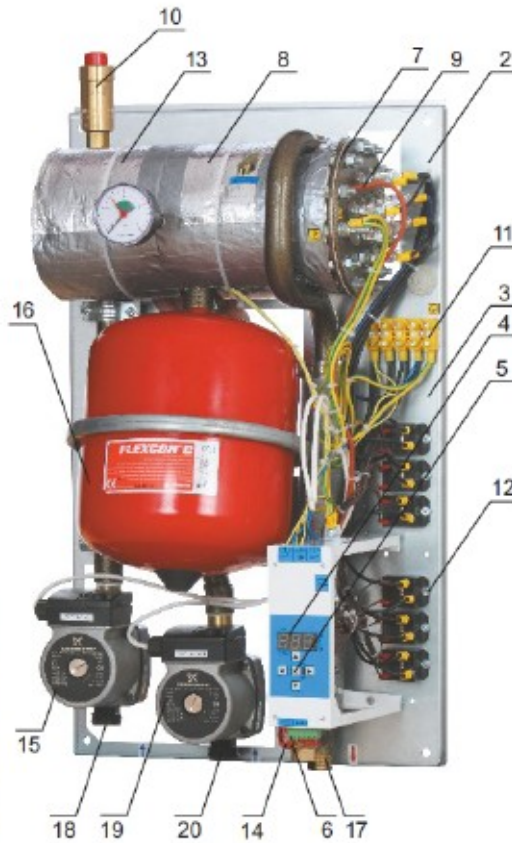
ELEMENTI TROVANTISI NELLA CALDAIA
