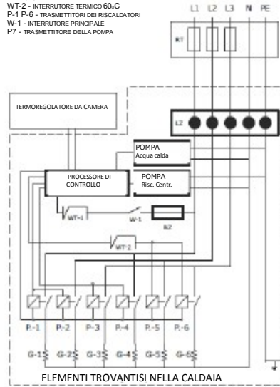
ELEMENTI TROVANTISI NELLA CALDAIA
