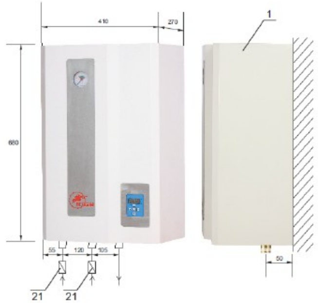
21 - Valvole di ritorno obbligatorie per il montaggio della caldaia
